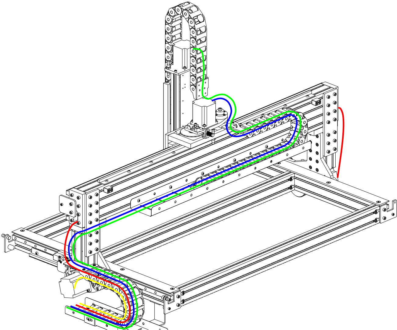
Motor Cables
